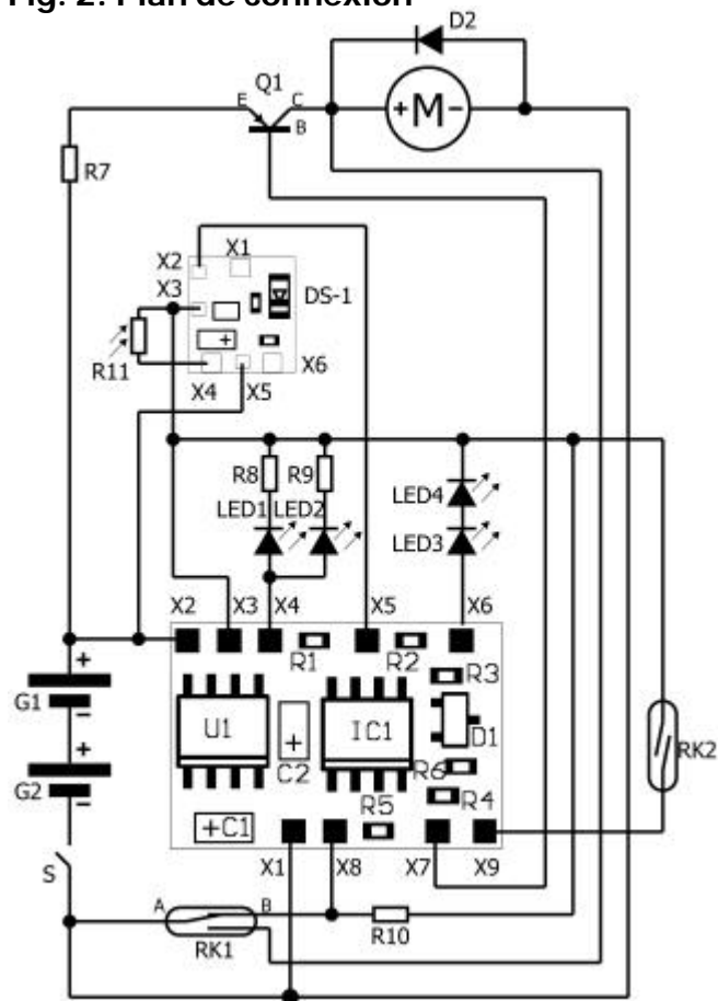
Fig. 2: Plan de connexion
