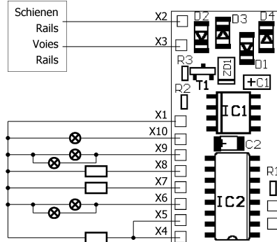
Fig. 1b: Anschluß bei Verwendung des Rückleiters X1 Connection when using the return conductor X1 Raccordement des fonctions vi la borne commune X1 Aansluiten bij gebruik van de retourleiding X1
