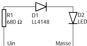
Fig. 1: Schaltplan
