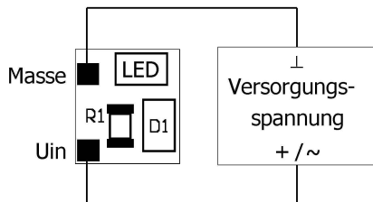
Fig. 2: Anschlußplan
