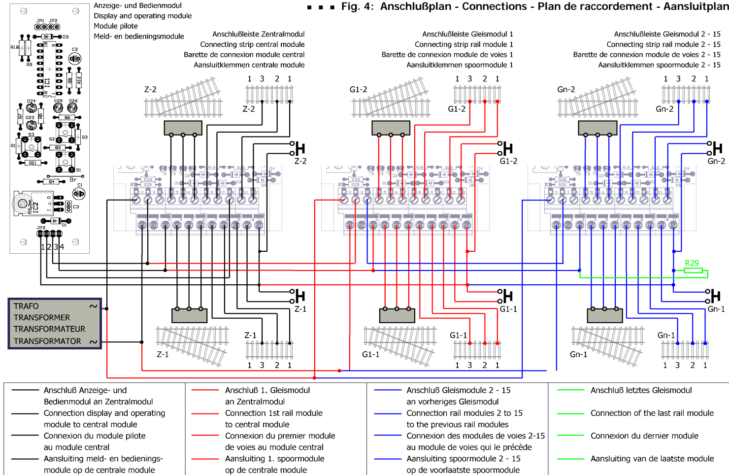
■ ■ Fig. 4: Anschlußplan - Connections - Plan de raccordement - Aansluitplan
